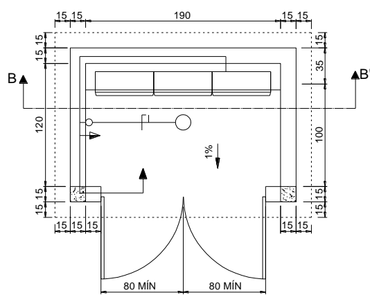
PLANTA BAIXA
