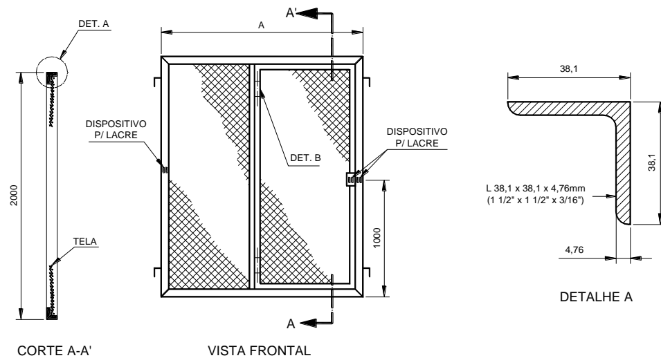
CORTE A-A'
